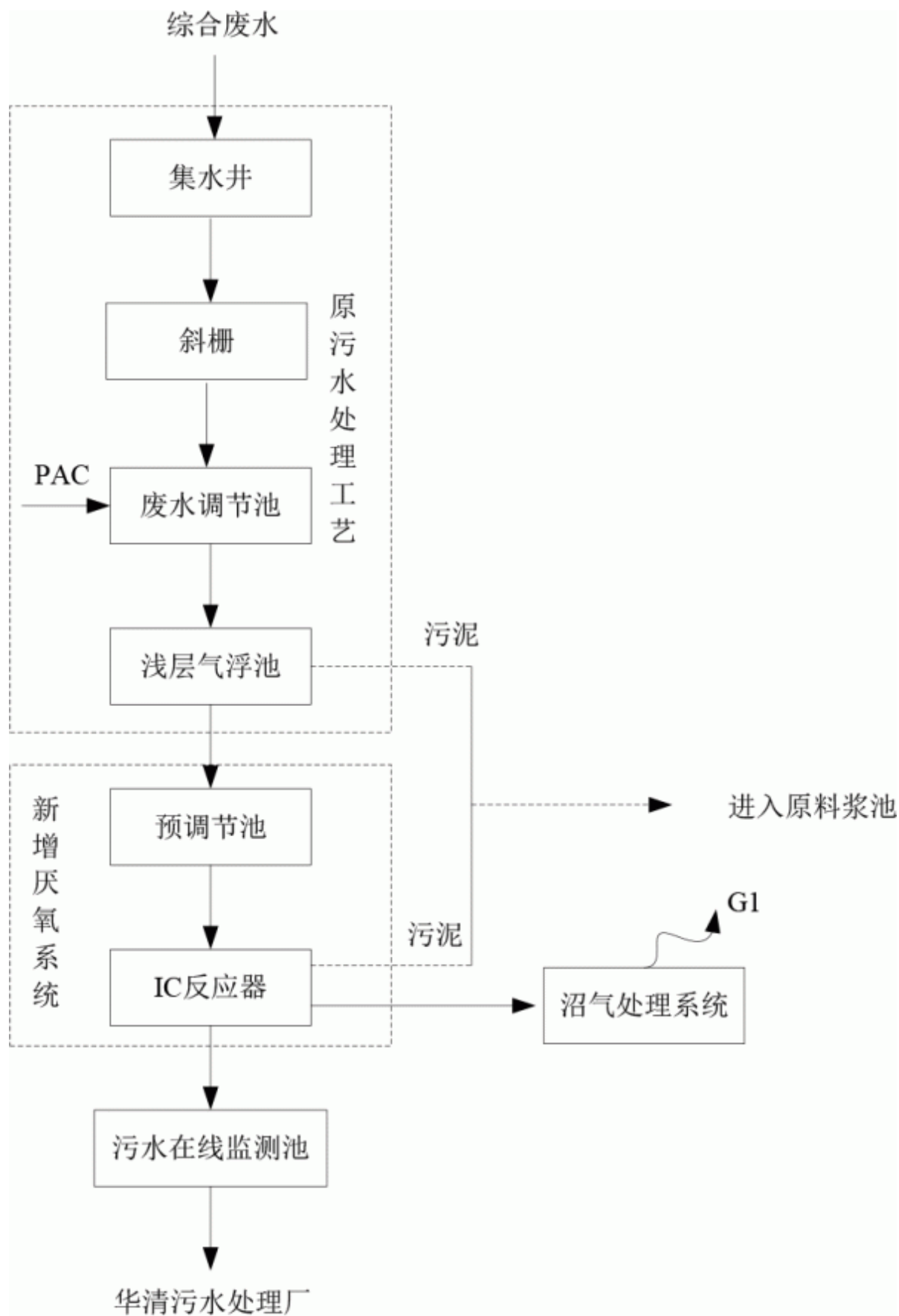
图 1 污水处理工艺流程图
